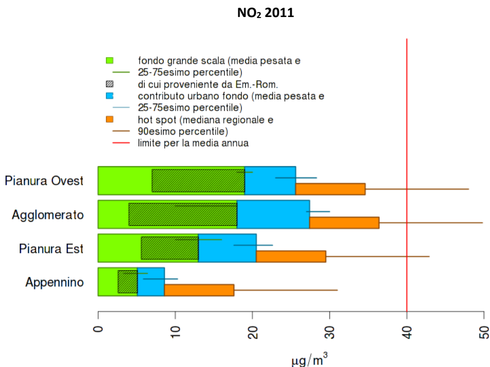
Figura 5.3.4 - Origine geografica dell'inquinamento da \text{NO}_x
